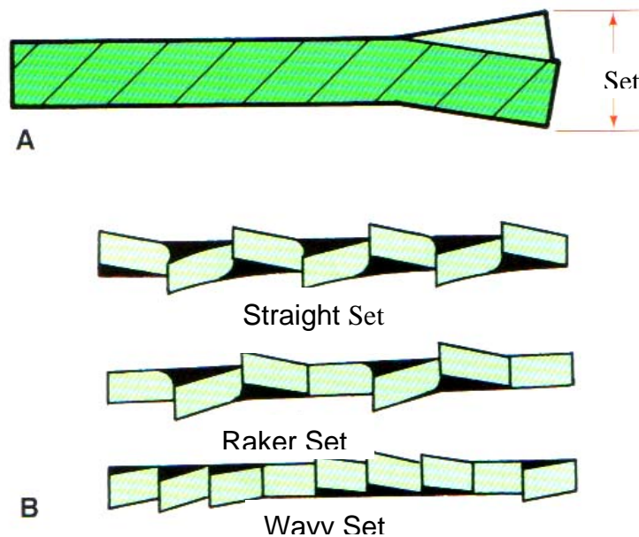
Fig. 3 Blade Set
